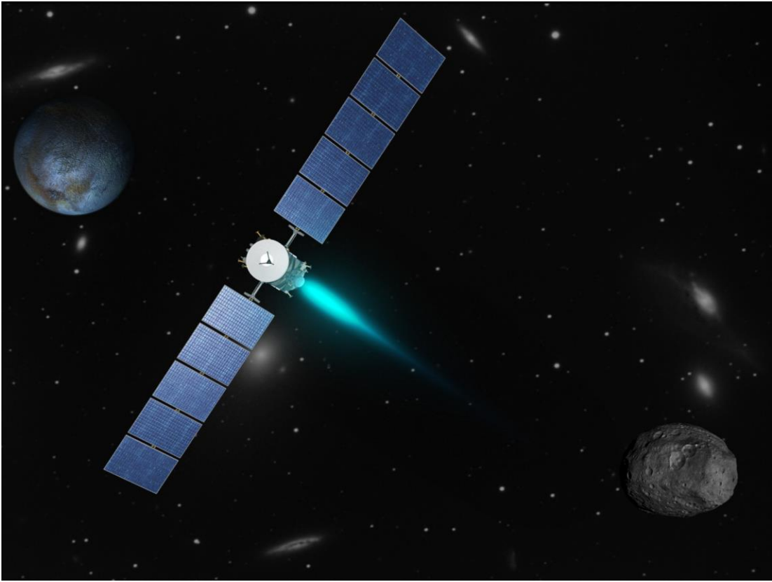
Dawn
